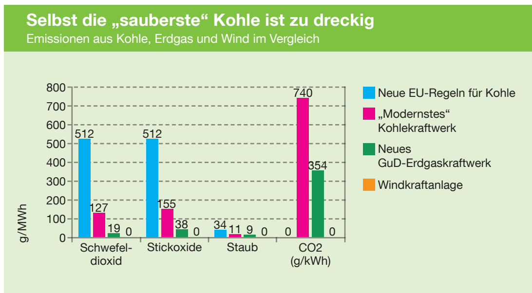
Abbildung 2: Die neuen EU-Luftverschmutzungsvorschriften für Kohlekraftwerke erlauben wesentlich höhere Emissionen als derzeit durch die bestmöglichen technischen Maßnahmen erreichbar wären, und mehr als 10-mal höhere Emissionen als ein neues gasbetriebenes Kraftwerk verursacht. 19
