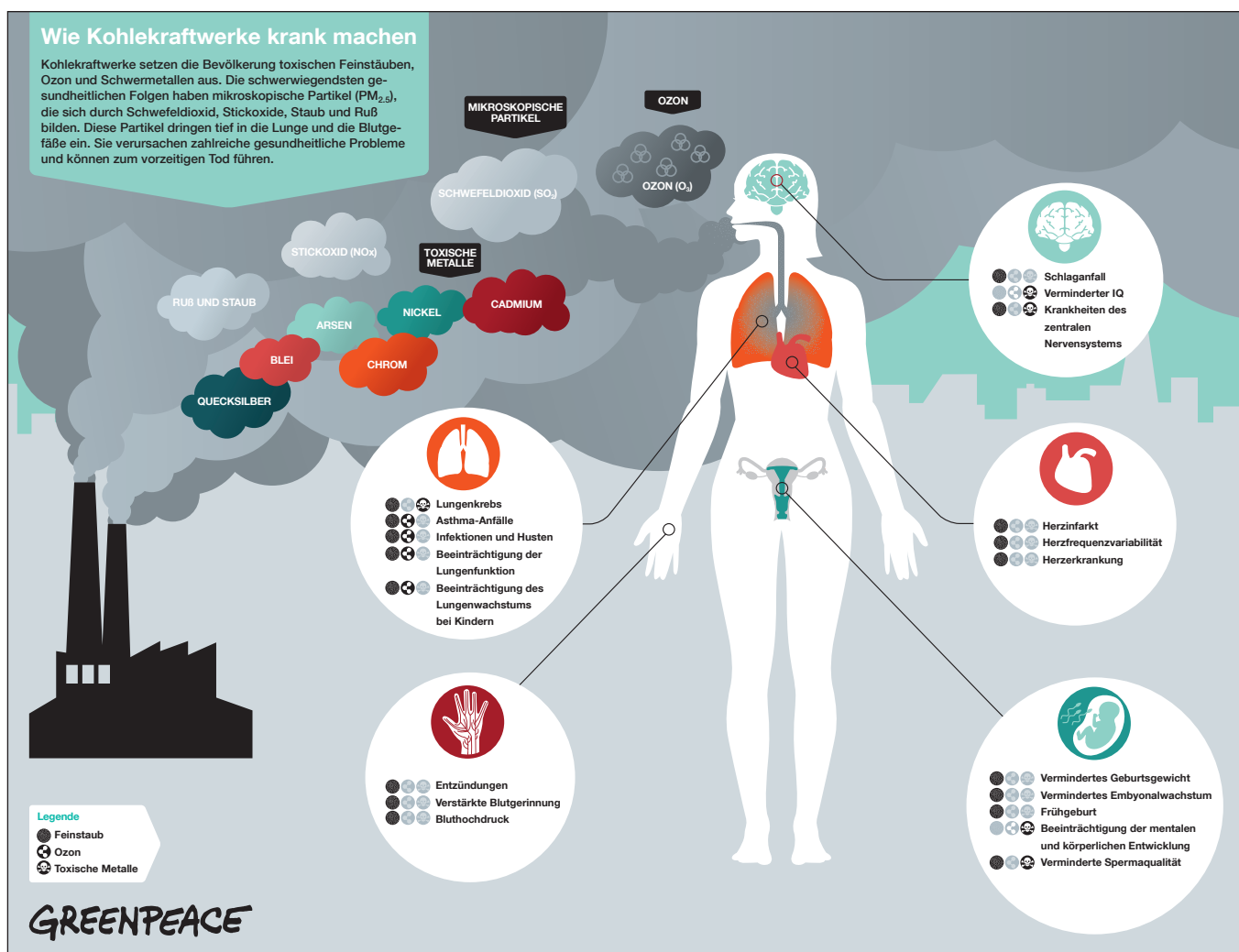
Abbildung 1: 18 Die Auswirkungen der Emissionen von Kohlekraftwerken auf den menschlichen Körper
